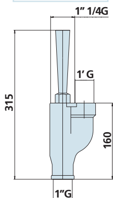
INJEKTOR 4"
